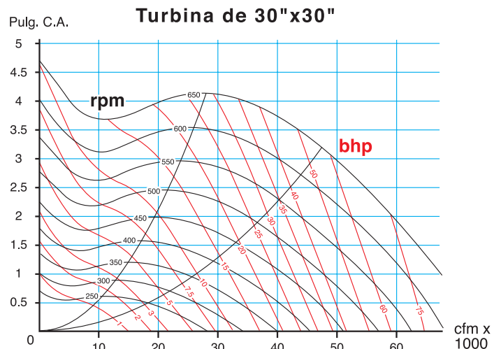
Curvas del ventilador, SNM
