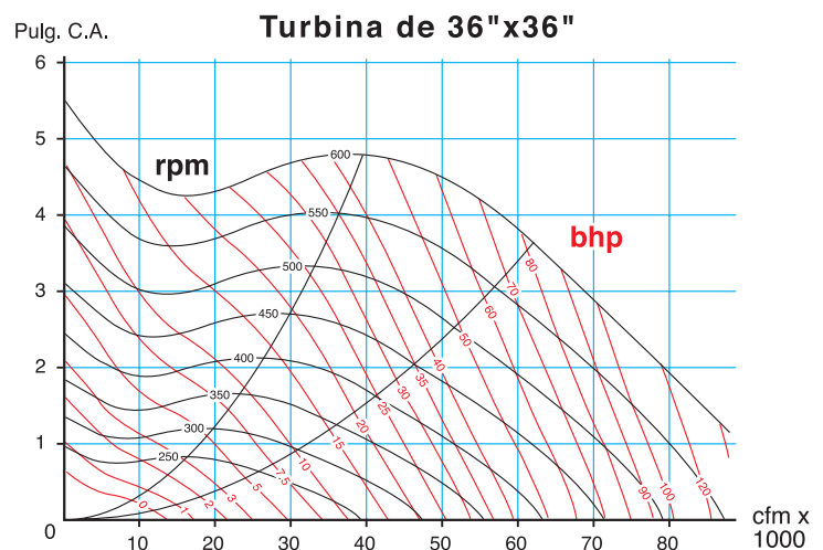
Curvas del ventilador, SNM
